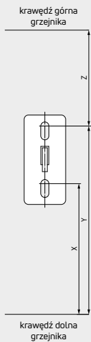
Rysunki schematyczne
